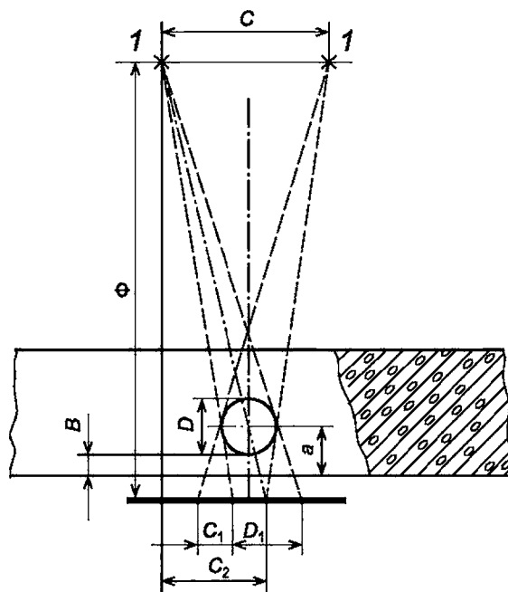
D — диаметр арматурного стержня; O_1 — проекция арматурного стержня; B — толщина защитного слоя; \Phi — фокусное расстояние; C — расстояние между первым и вторым положением источника; C_1 — смещение проекций арматурного стержня на пленку; C_2 — расстояние от оси проекции стержня до прямой, проходящей через источник перпендикулярно поверхности преобразователя излучения; a — расстояние от поверхности конструкции до центра арматуры; 1 — источник излучения
