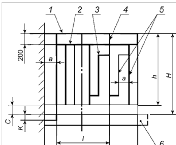
Рисунок А.3 - Перильное ограждение лестничного марша с наклонными промежуточными ограждающими элементами
