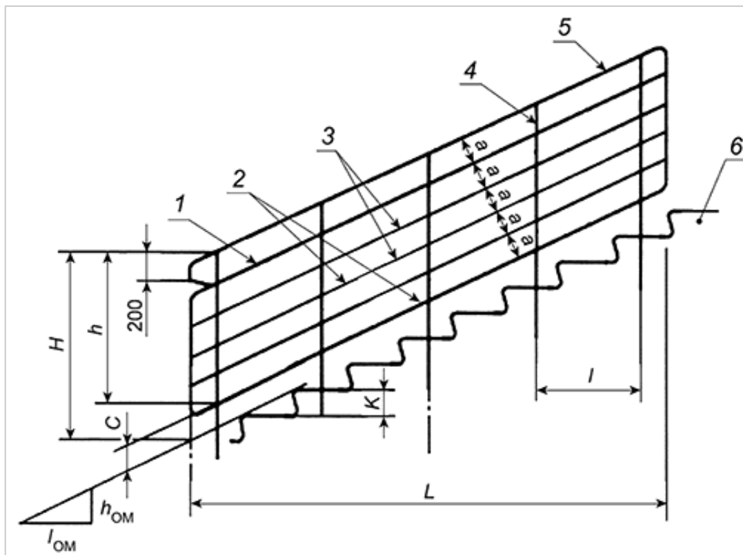
Рисунок А.2 - Экранные и комбинированные ограждения лестничных маршей
