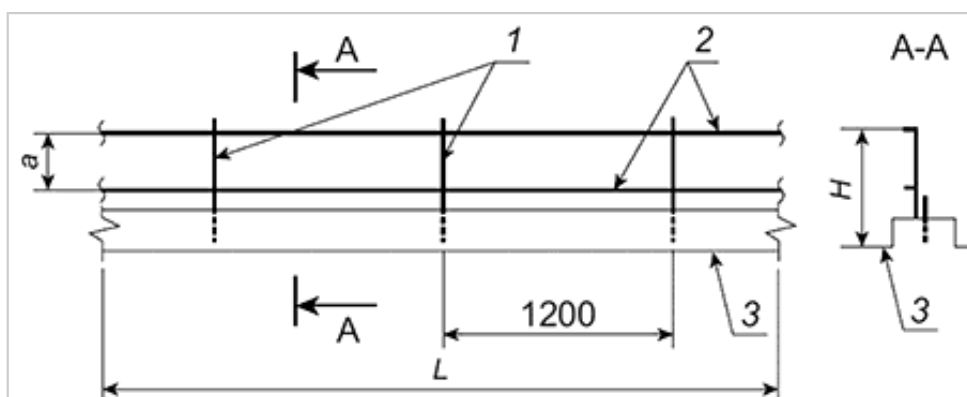
Рисунок А.8 - Ограждения крыш без парапета
