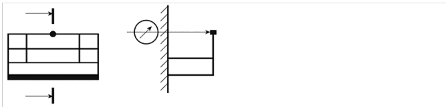
Рисунок 1 - Схема приложения статической нагрузки при испытании прочности ограждений
