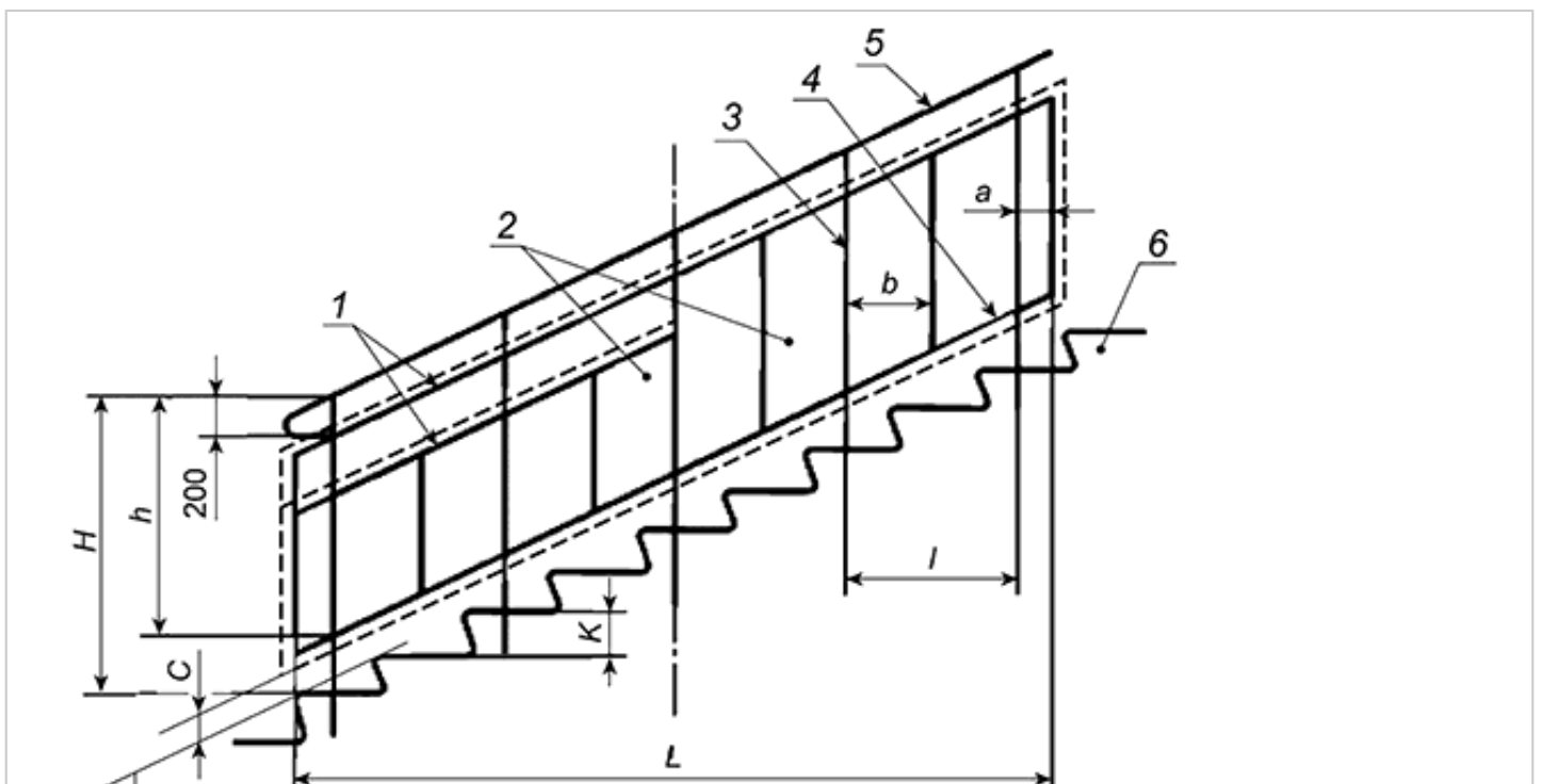
Рисунок А.1 - Решетчатые ограждения лестничных маршей
