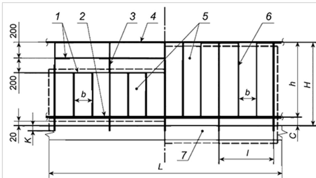
Рисунок А.6 - Решетчатые ограждения балконов
