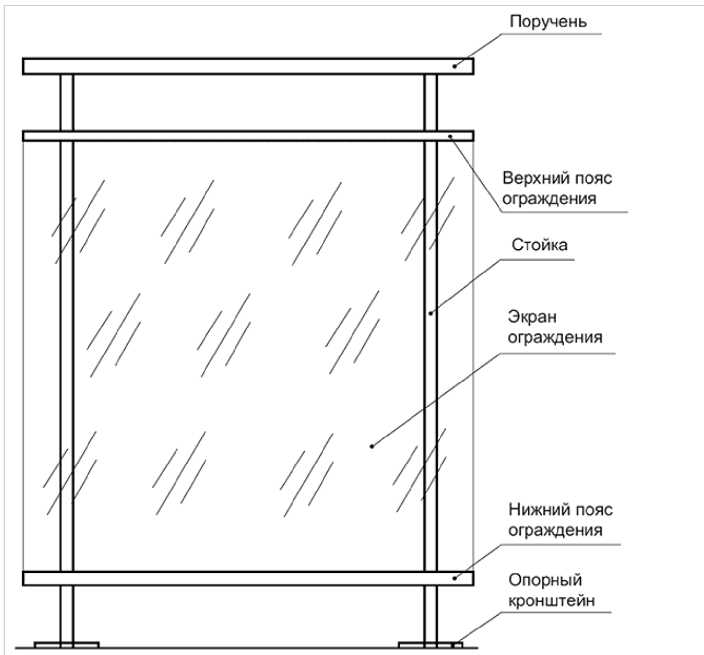
Рисунок Б.3 - Вариант светопрозрачного экранного ограждения с креплением к перекрытию
