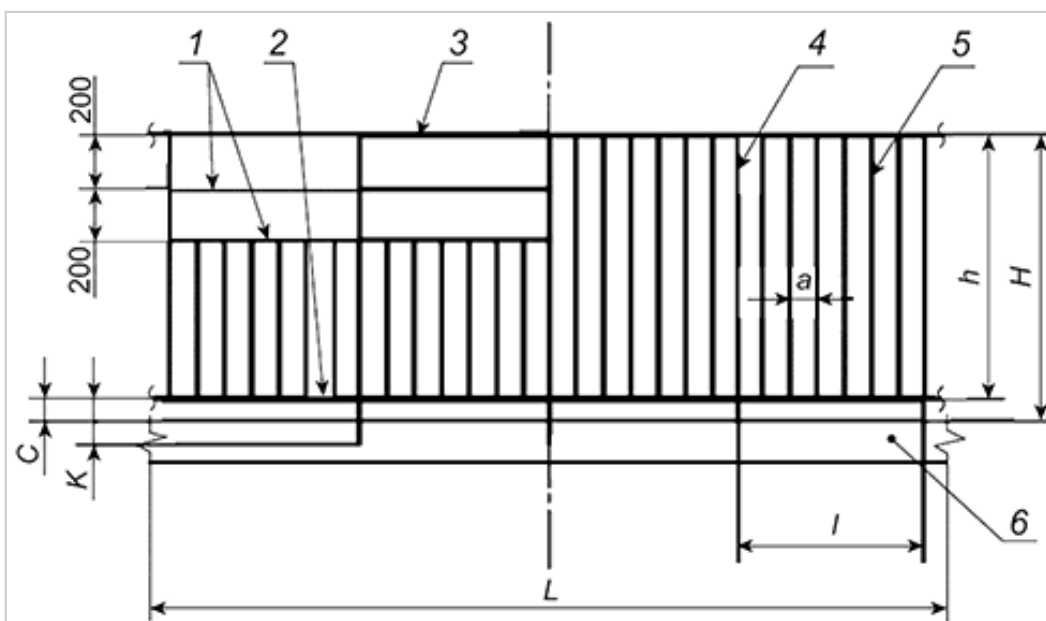
Рисунок А.5 - Экранные и комбинированные ограждения лестничных площадок
