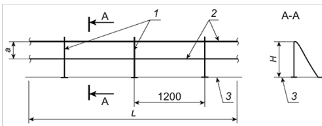
Рисунок А.7 - Экранные и комбинированные ограждения балконов
