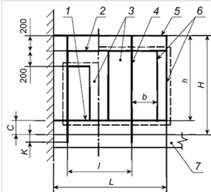
Рисунок А.4 - Решетчатые ограждения лестничных площадок
