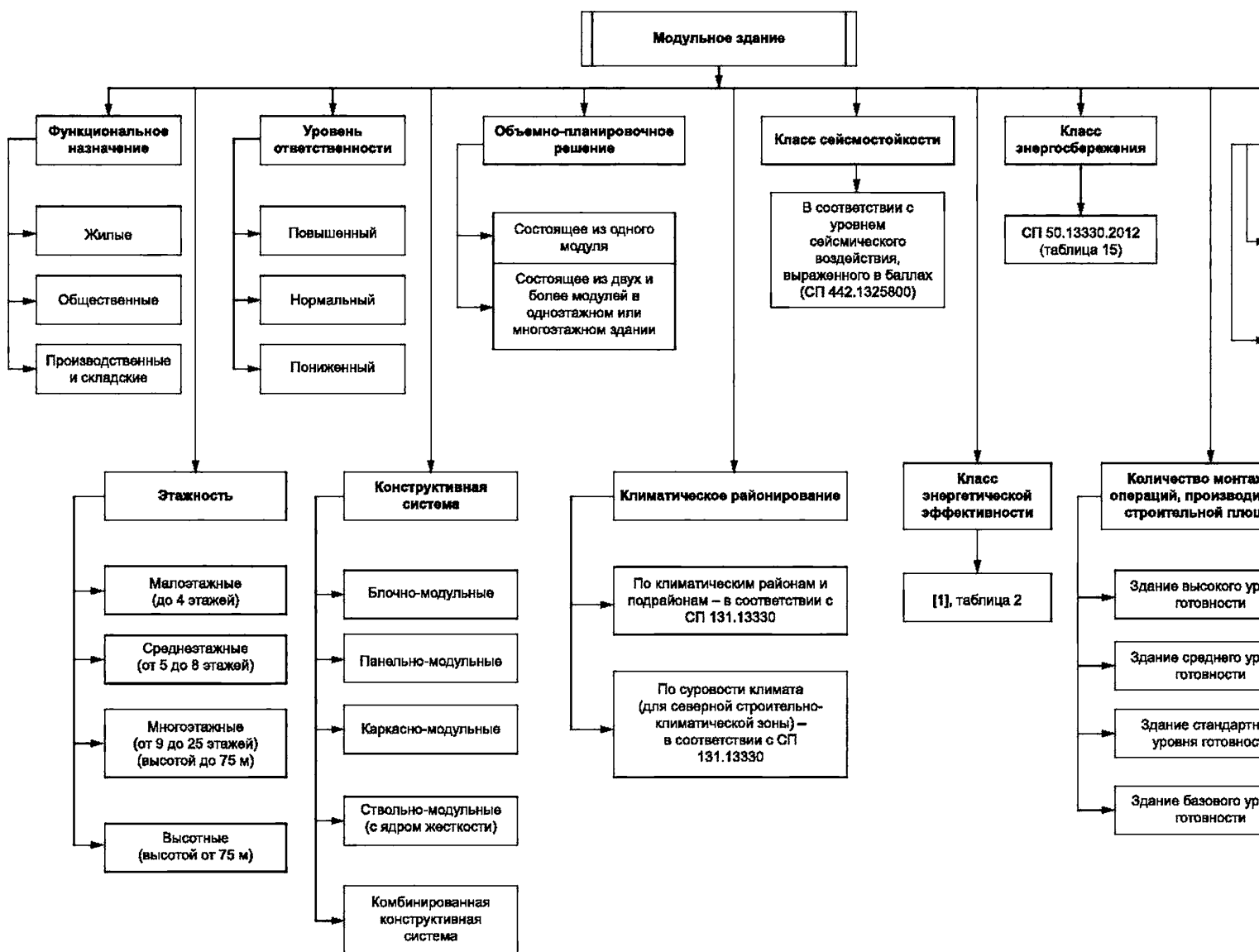
Рисунок А. 1 – Классификация модульных зданий
