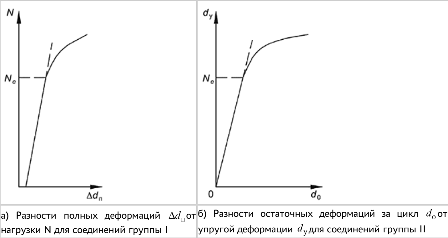
Рисунок Б.3 - Диаграмма зависимости деформаций
