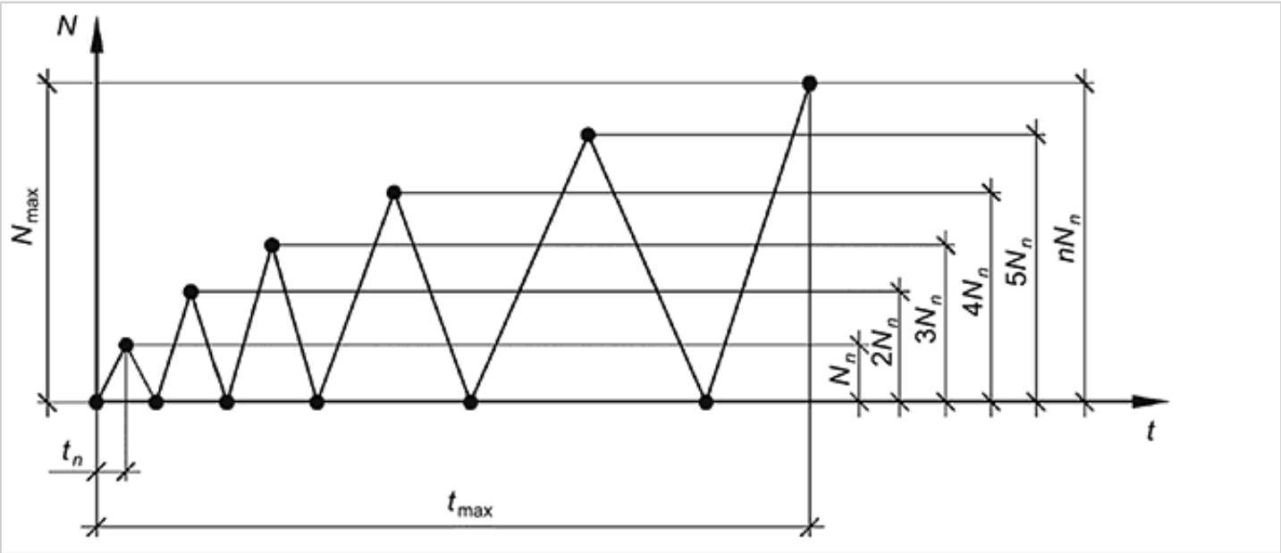
Рисунок Б.1 - Диаграмма приложения на образец непрерывно возрастающей нагрузки
