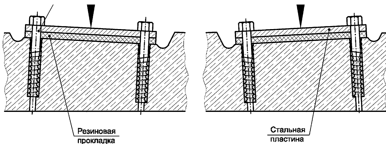
Рисунок 18 — Схема измерения электрического сопротивления шпалы
