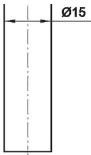
Рисунок 19 — Схема шаблона для контроля прямолинейности внутреннего канала в дюбеле
