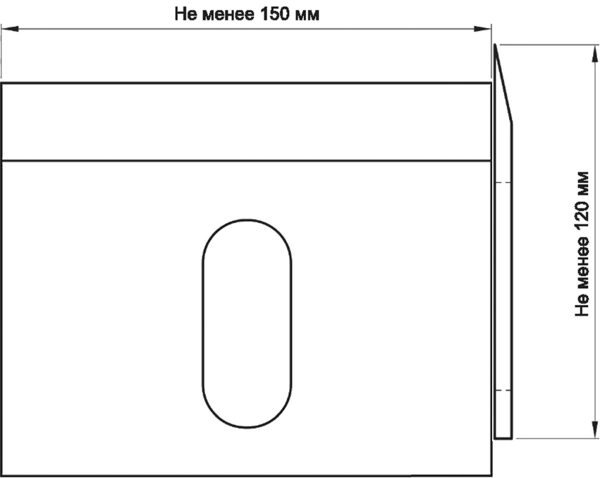
Рисунок 9 – Металлический шаблон
