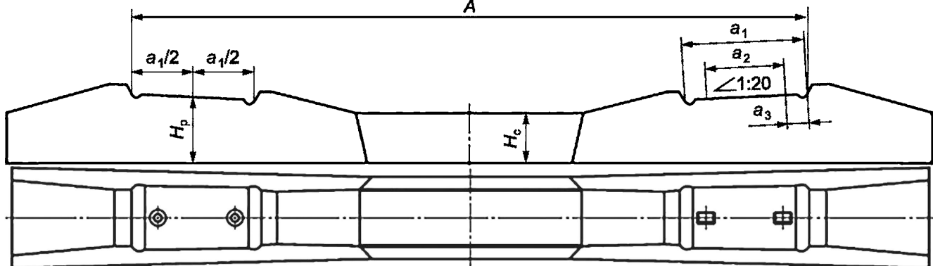
Рисунок 3 — Схема шпал типа III
