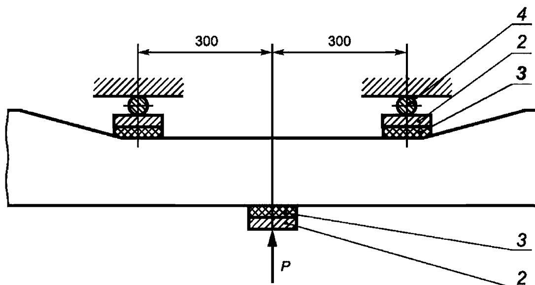
а — в подрельсовом сечении
