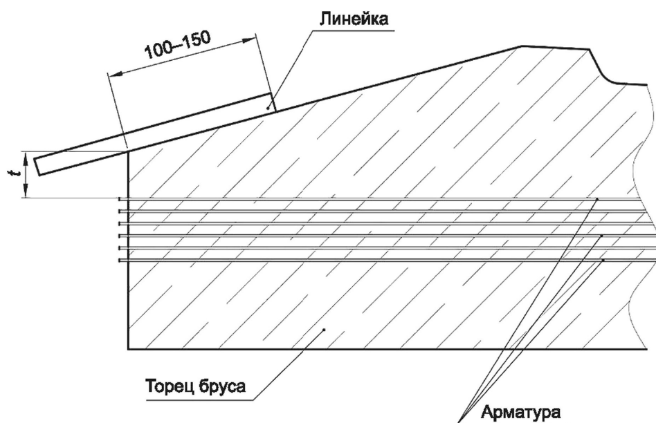
Рисунок 17 — Схема определения толщины t защитного слоя бетона
