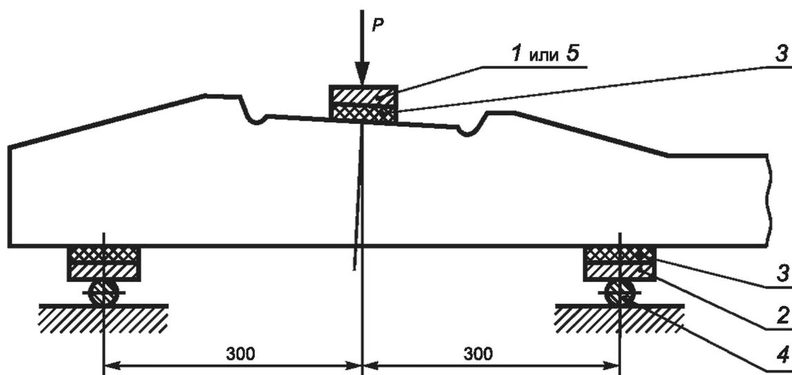
а — в подрельсовом сечении
