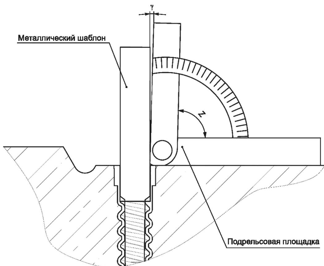
Рисунок 13 — Схема контроля угла наклона дюбеля y
