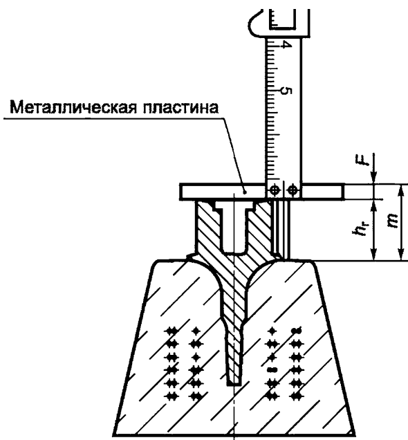
Рисунок 14 — Схема контроля высоты головки анкера
