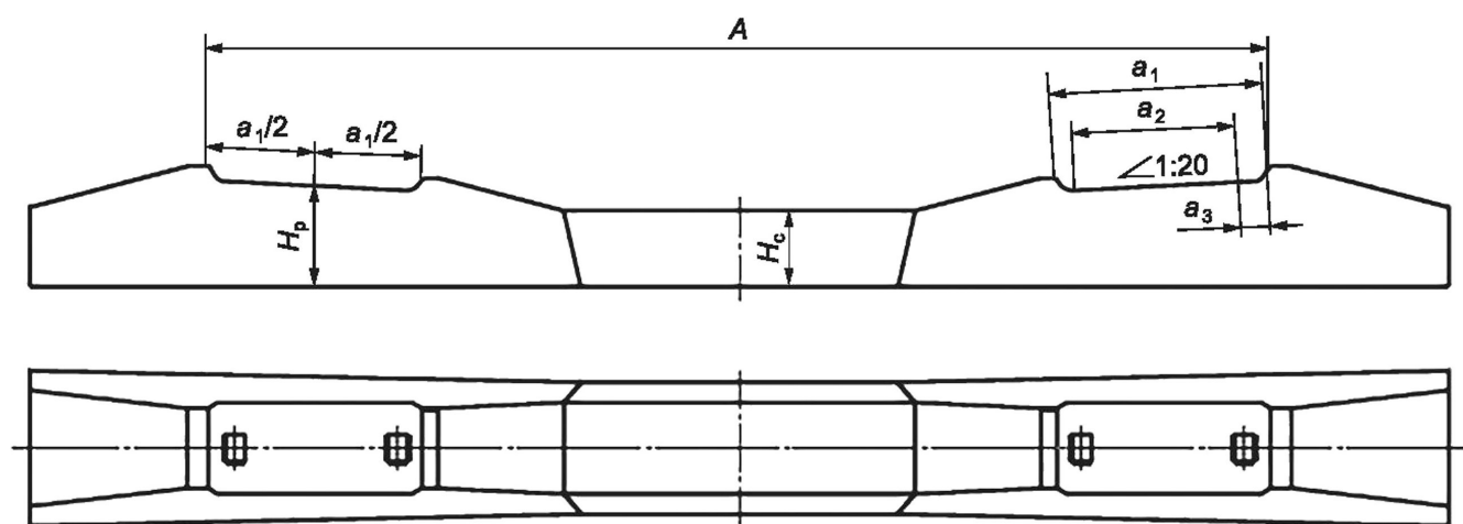
Рисунок 1 — Схема шпал типа I
