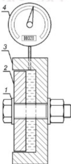
1 — болтокомплект; 2 — поршень; 3 — корпус; 4 — манометр или индикатор усилия
